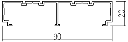
เฟรมข้างบานเลื่อนยูโร
