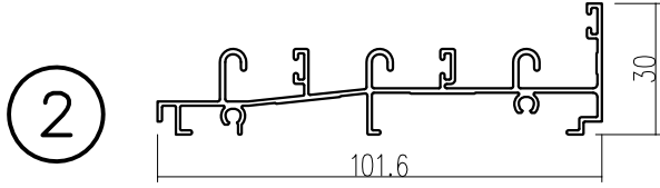
เฟรมล่างบานเลื่อน3รางธรณีต่ำ
