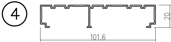
เฟรมข้างบานเลื่อน3ราง
