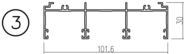
เฟรมบนบานเลื่อน3ราง
