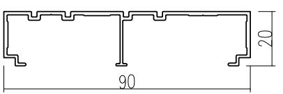
เฟรมข้างบานเลื่อน
