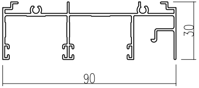
เฟรมบนบานเลื่อน
