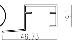
ตบธรณี บานเลื่อนยูโร
