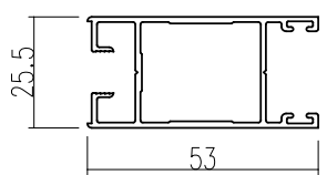
เสากูญแจ/เกี้ยว 53 มม.
