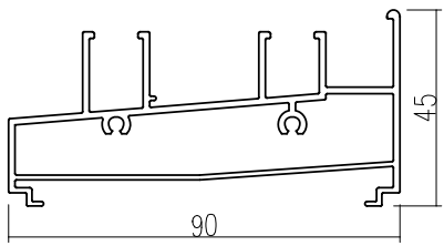
เฟรมล่างบานเลื่อนยูโร(แบบถอดวาง)
