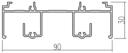
เฟรมบนบานเลื่อนยูโร
