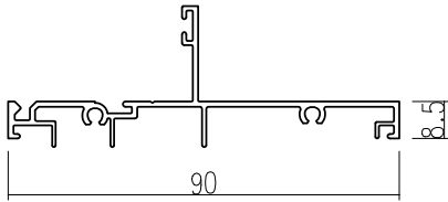
ตบเฟรมข้างบานตาย(บานเลื่อน)
