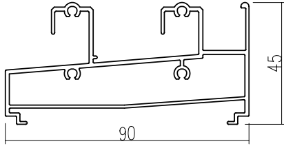
เฟรมล่างบานเลื่อนยูโร
